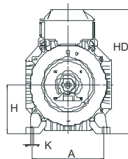
Foot-mounted motor IM 1001, B3
