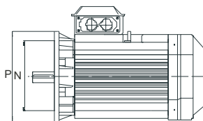
Flange-mounted motor IM 3001, B5
