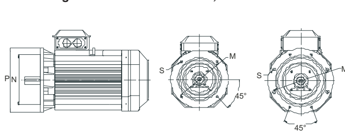
Flange-mounted motor IM 3001, B5
