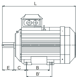
Foot-mounted motor IM 1001, B3
